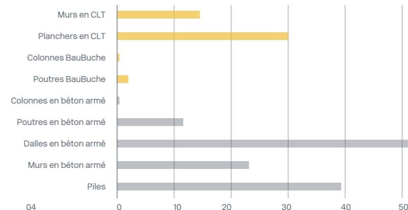
Carbone incorporé dans le bâtiment en kgCO 2 e/m 2
